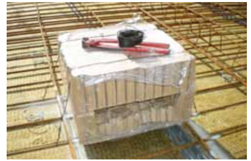
La fixation des réservations en carton nid d'abeilles sur le treillis est faite avec du fil de fer.
